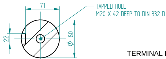
Przekrój A-A 1:3
